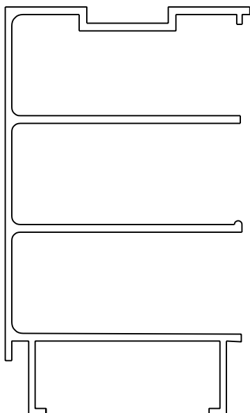
PERFIL NRO. 190 ZOCALO PASACABLES M-2549 1.029 KG./ML.
