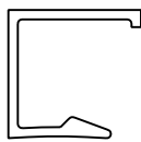
PERFIL NRO. 193 CONTRAVIDRIO LARGO M-2552 0.132 KG./ML.
