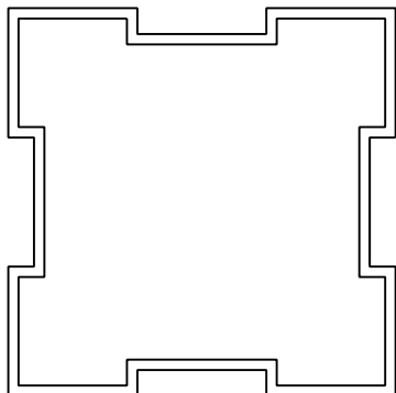
PERFIL NR. 195 COLUMNA M-2554 0.645 KG./ML.
